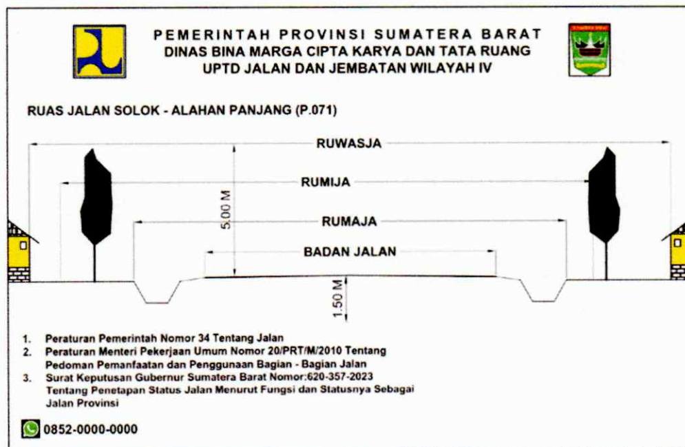
Gambar 3.1 Papan informasi ruas jalan
